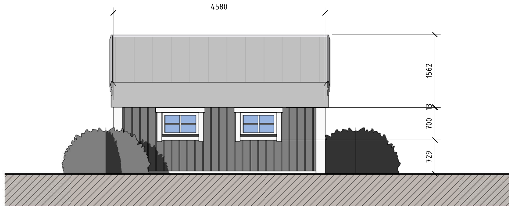
Fasad mot Norr SKALA 1 : 50
